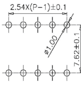
P.C.B LAYOUT
